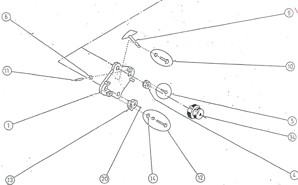
ENSEMBLE ROULEAU
